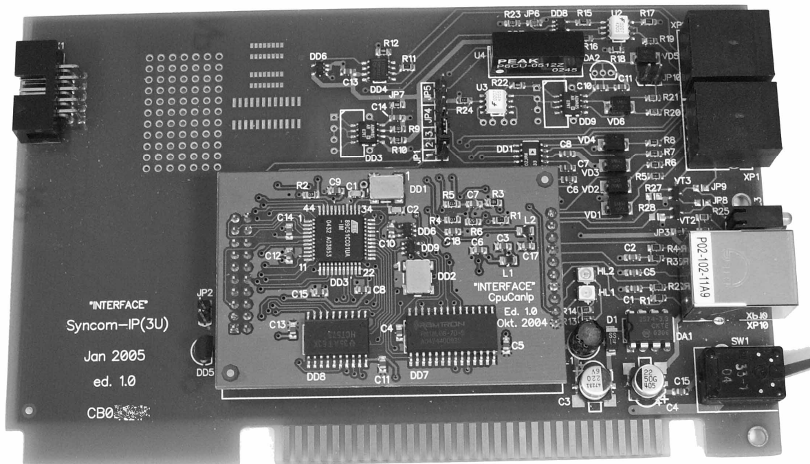
Рис. 1. Внешний вид контроллера “Синком-IP(3U)”.
